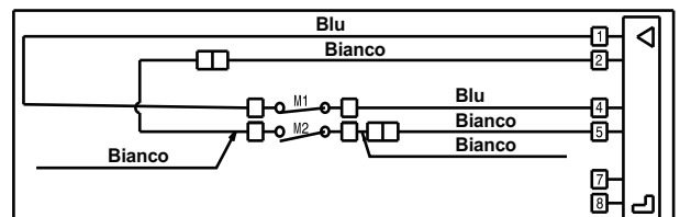
Cablaggio Micro / Microswitches Wiring
