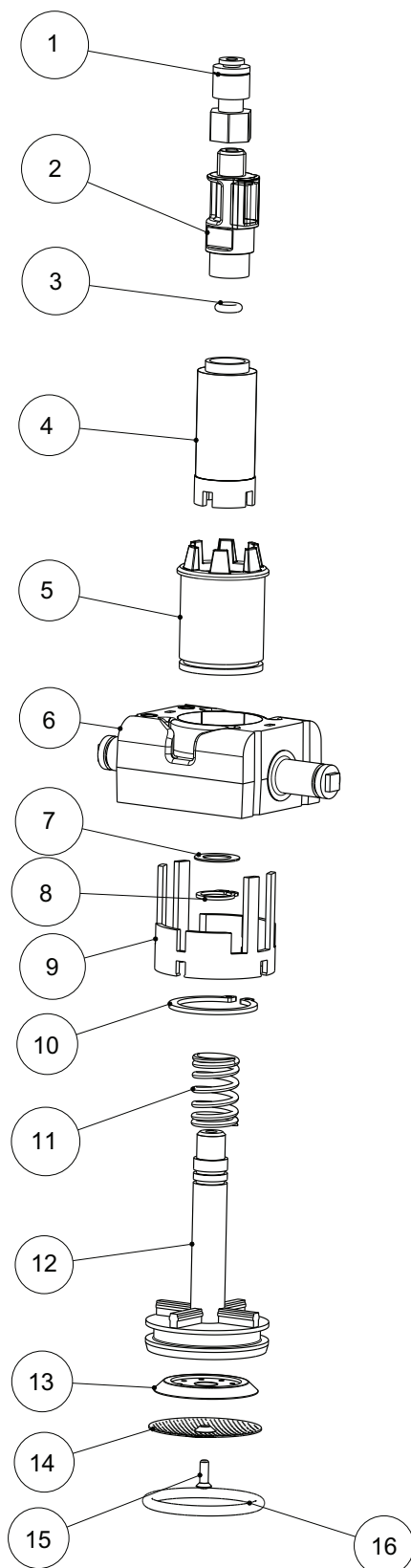
Пистон с верхним поршнем в сборе (поз.5)
