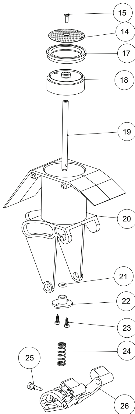
Заварная камера (поз.7)
